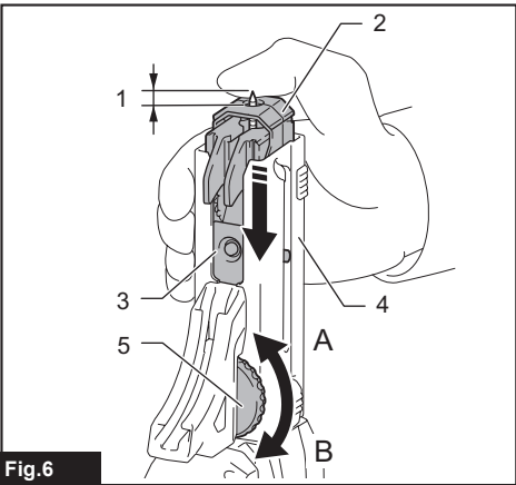
► 1. Aprox. 6 mm (1/4") 2. Base del tope 3. Surtidor 4. Estuche 5. Selector de ajuste
