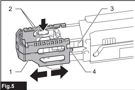
► 1. Base del tope 2. Palanca 3. Placa 4. Estuche
